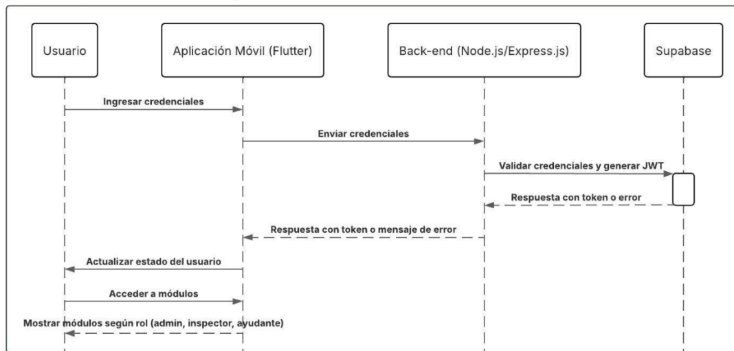
Diagrama de Secuencia de Autenticación de Usuario.
